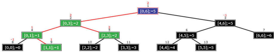
Рис. 2.8 ❖ Дерево сегментов массива A = \{18, 17, 13, 19, 15, 11, 20\} и \text{RMQ}(1, 3)
