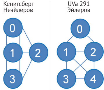
Рис. 4.41 ❖ Эйлеров граф
