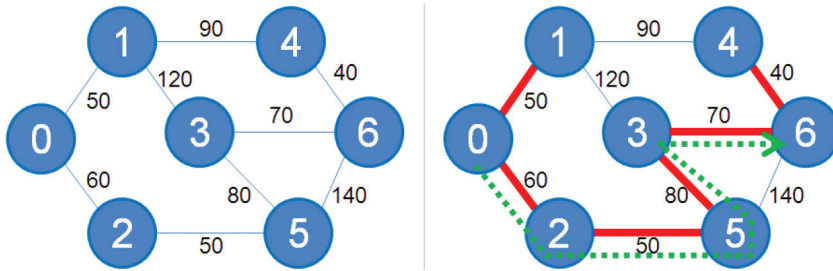
Рис. 4.16 ❖ Минимакс (UVa 10048 [47])
