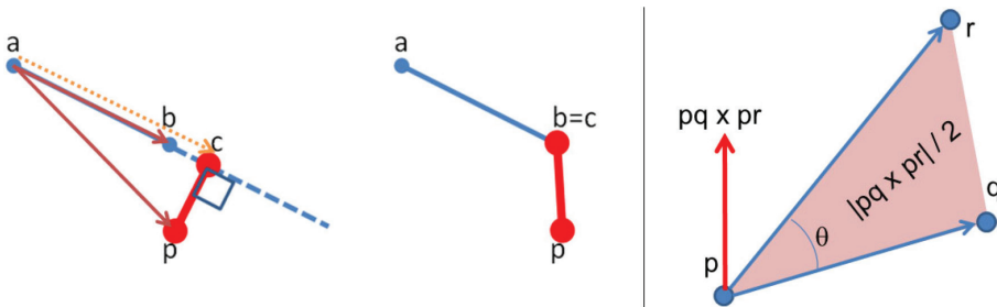
Рис. 7.2 ❖ Расстояние до прямой (слева) и до отрезка (в середине); векторное произведение (справа)
