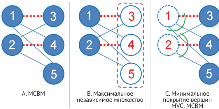
Рис. 4.43 ❖ Варианты МСВМ
