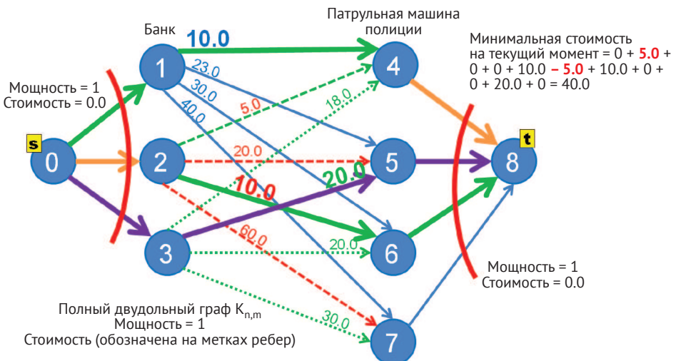
Рис. 9.5 ❖ Пример тестового варианта при решении задания UVa 10746: три паросочетания с минимальной стоимостью = 40
