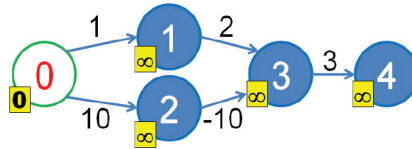
Рис. 4.18 ❖ Вес -ve
